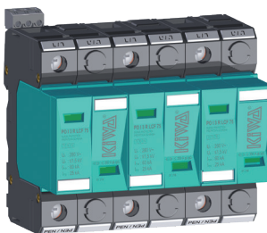
PO I 3 R LCF 75kA
