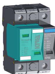
PO I 1+1m LCF 50kA
