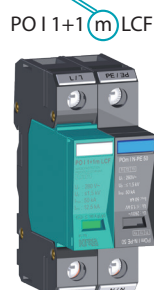
PO I 3+1 m LCF
