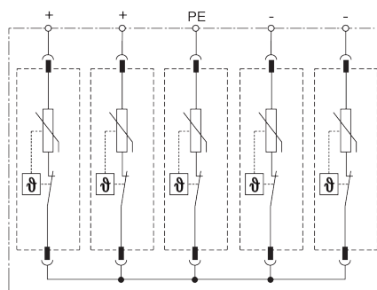
PO I 5 PV 600V DC Y 2-okr. PO I 5 PV 1000V DC Y 2-okr.
