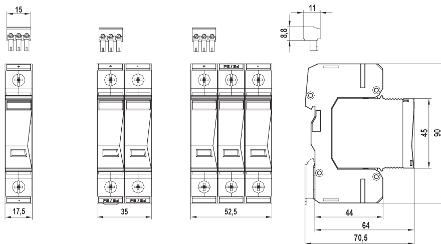
PO II 1 R PV 100V DC PO II 2 R PV 100V DC PO II 3 R PV 200V DC
